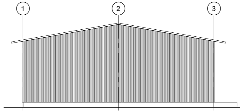
3 South 1 : 150
