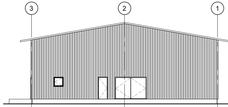
2 North 1 : 150
