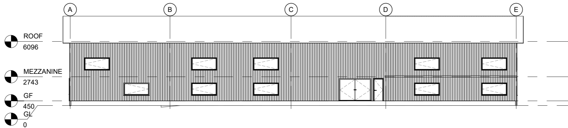
2 West 1 : 150
