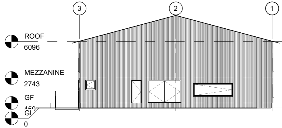
1 North 1 : 150
