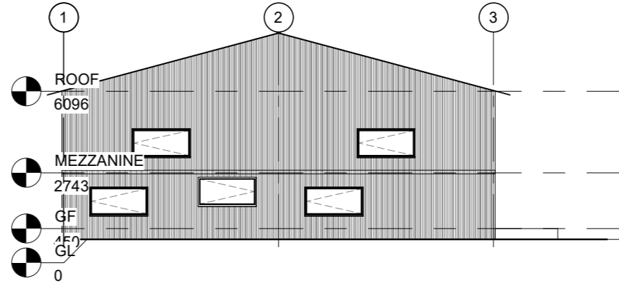
3 South 1 : 150
