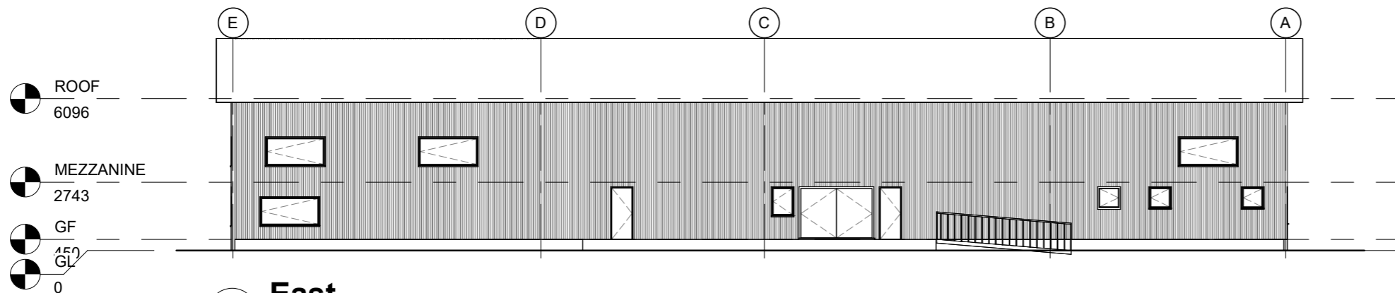
4 East 1 : 150
