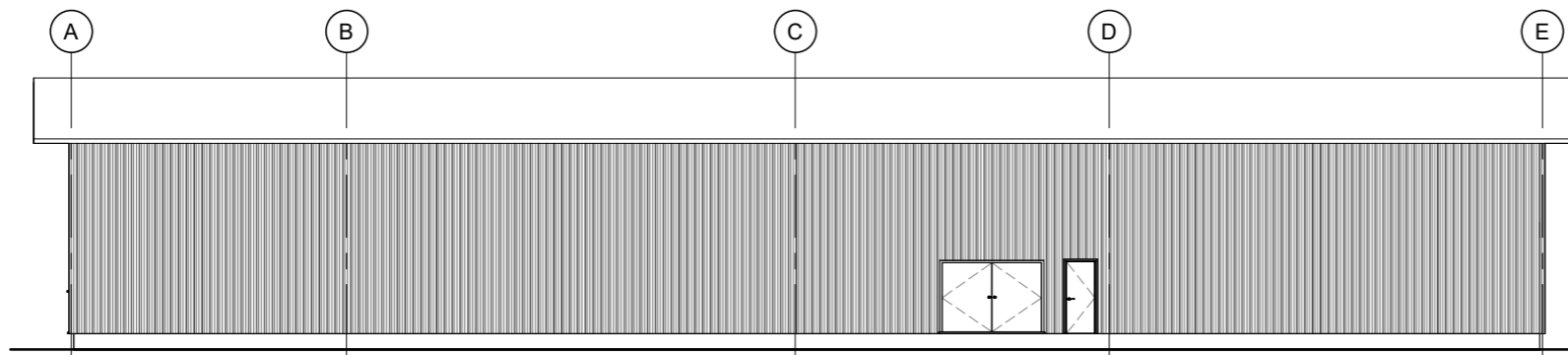
4 West 1 : 150
